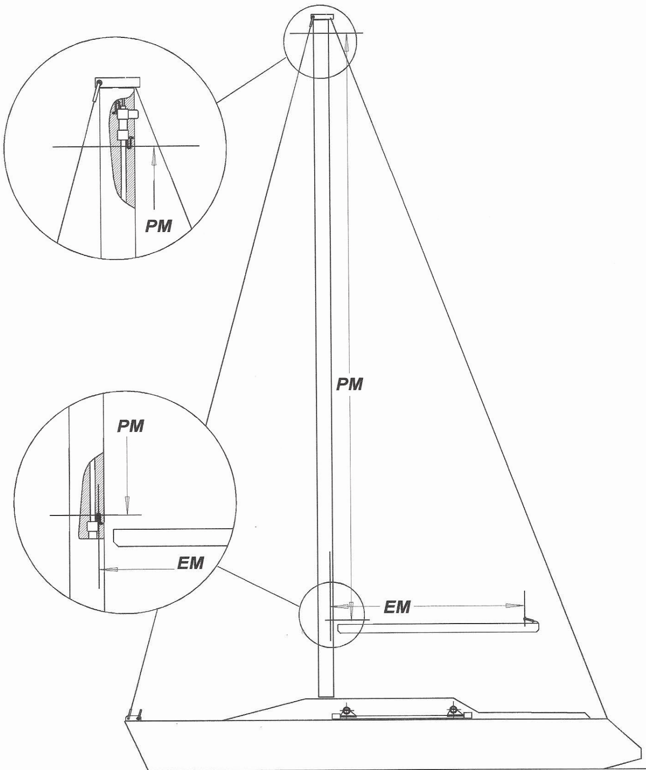
Prise de mesures pour grand-voile enrouleur
