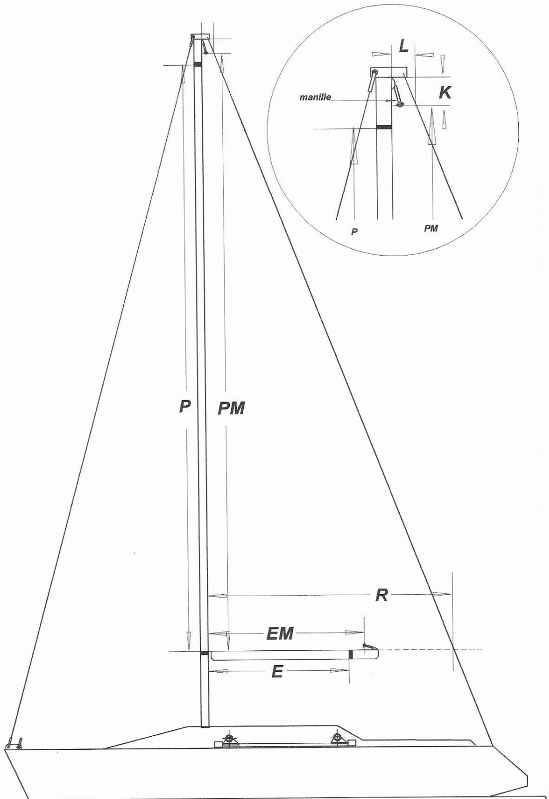
Prise de mesures pour grand-voile
